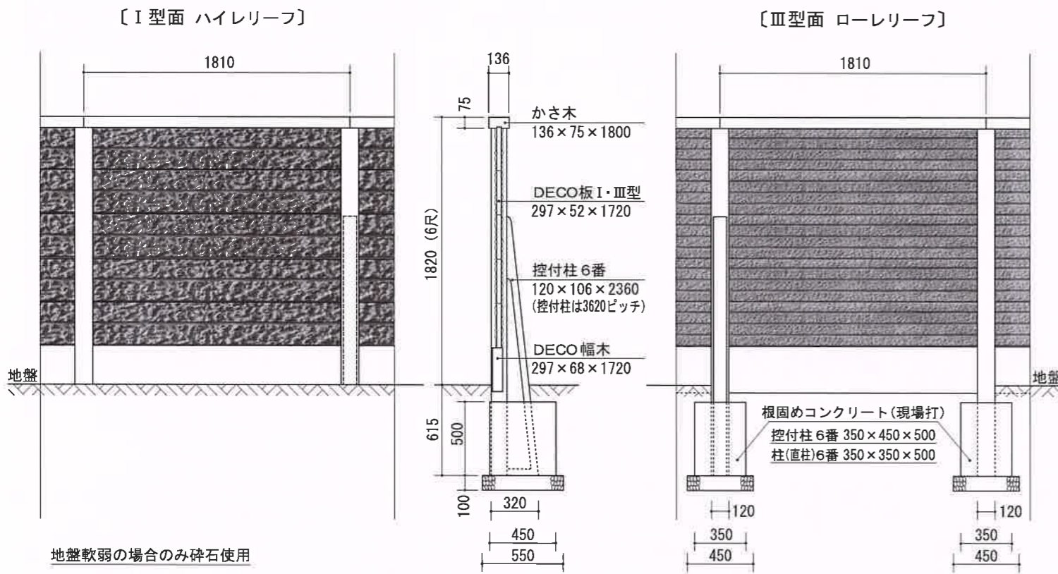
DECO塀 I・III型 地上高1820(6尺) 標準型
